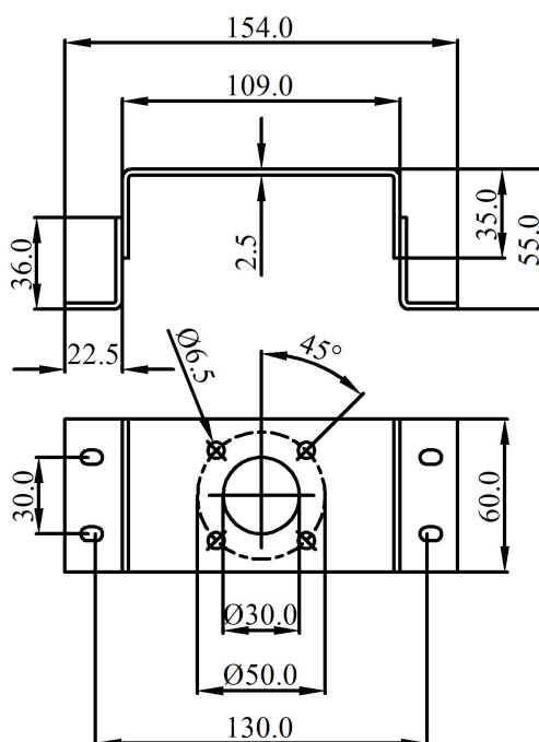
Монтажный кронштейн прямого хода с дистанционной передачей
