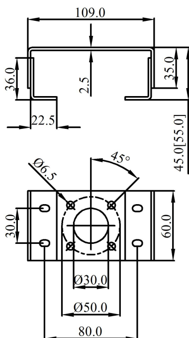
Обычный монтажный кронштейн с прямым ходом
